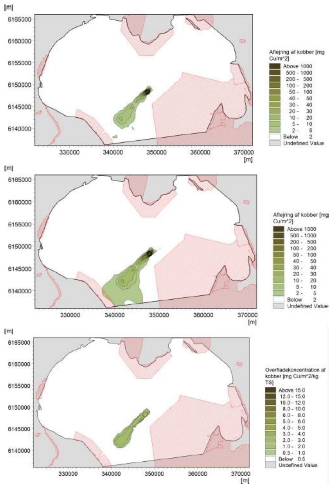
Figur 5-12. Aflejring af kobber efter første års klapning og ved brug af klappads Kb. Øverst: total mængde aflejret kobber (mg Cu/m 2 ) efter år 1. Midt: total mængde aflejret kobber (mg Cu/m 2 ) efter år 2. Nederst: Overfladekoncentration i de øverste 5 mm sediment (mg Cu/kg TS) /66/.
