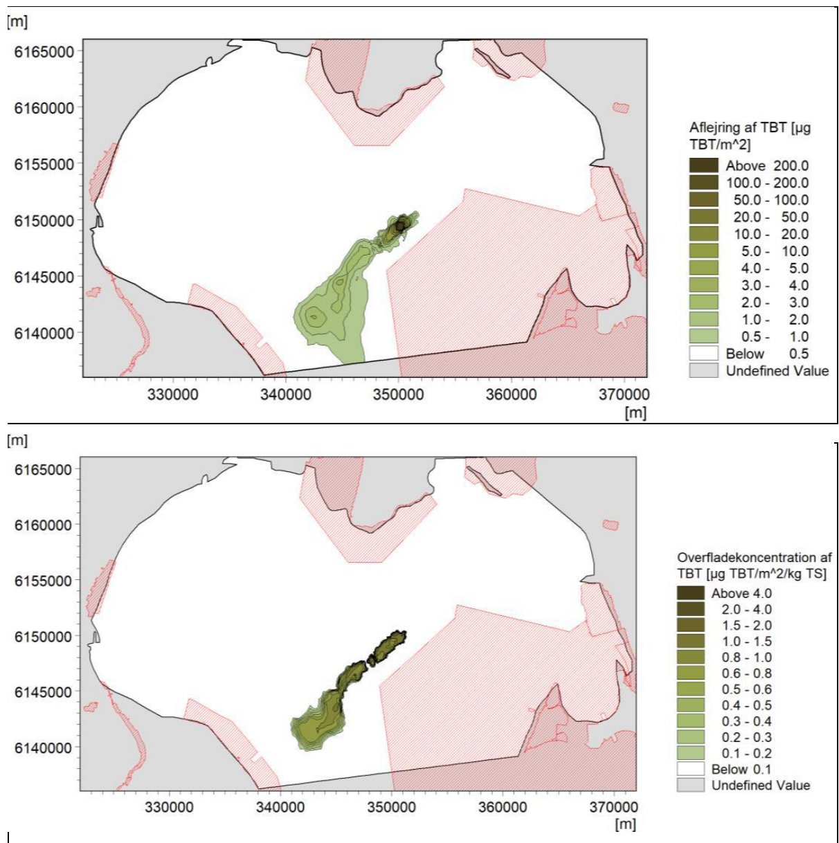
Figur 5-10. Aflejring af tributyltin (TBT) efter første års klapning og ved brug af klapplads Ka. Øverst: total mængde aflejret TBT ( \mu\text{g TBT}/\text{m}^2 ). Nederst: Overfladekoncentration ( \mu\text{g TBT}/\text{kg TS} ) i de øverste 2,5 mm sediment /66/.
