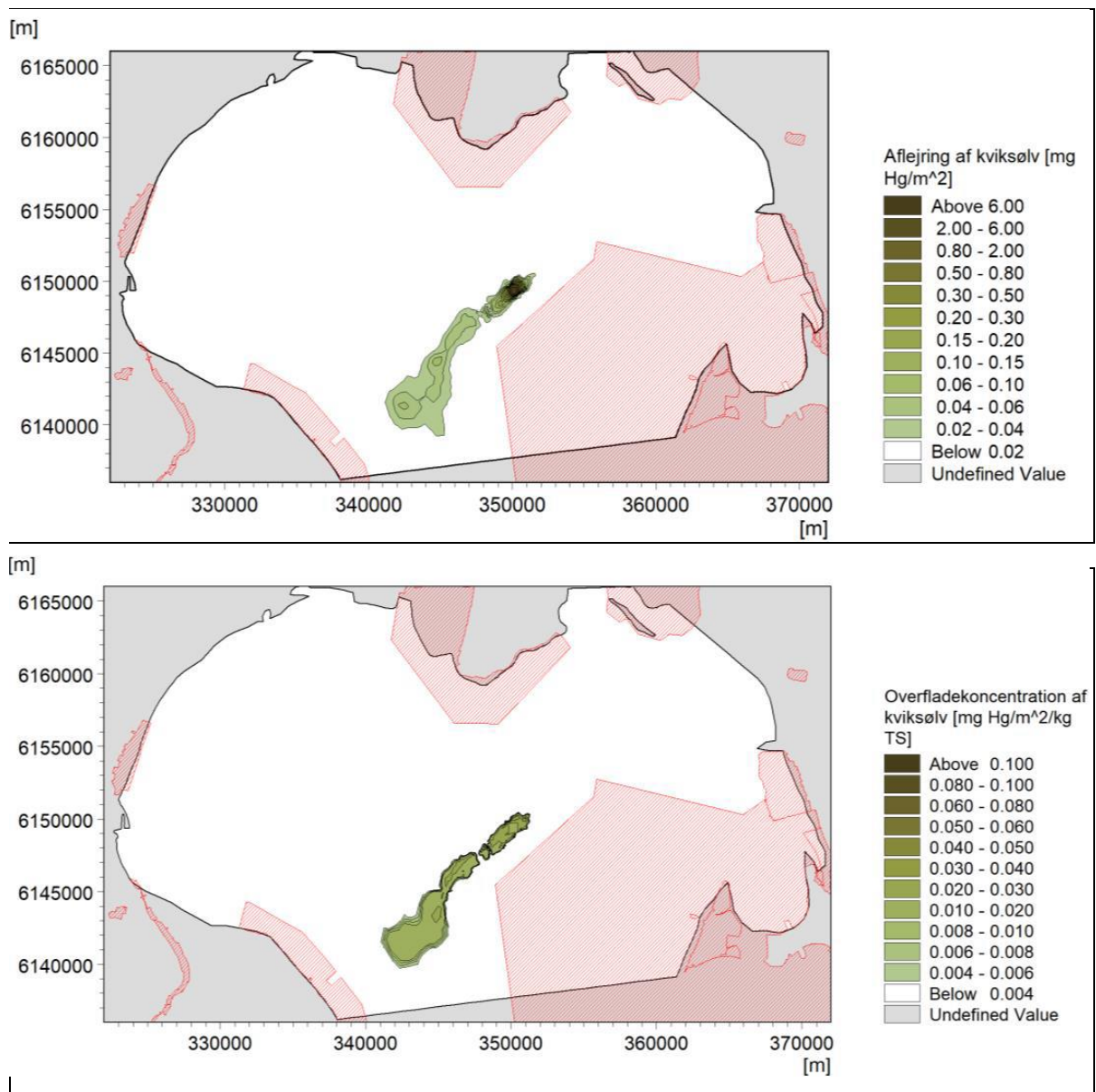
Figur 5-6. Aflejring af kviksølv efter første års klapning og ved brug af klapplads Ka. Øverst: total mængde aflejret kviksølv (mg Hg/m²). Nederst: Overfladekoncentration (mg Hg/kg TS) i de øverste 2,5 mm sediment /66/.
