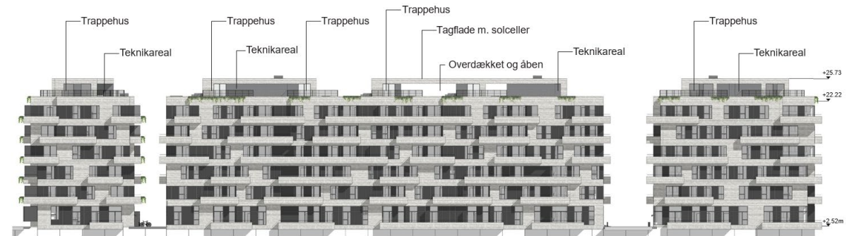
Facade mod Nord - Sundkaj
