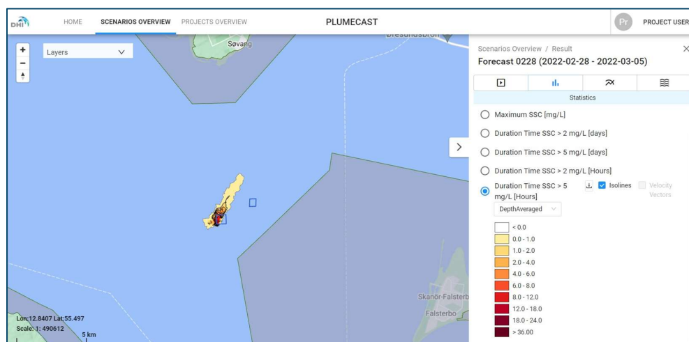
Figur 5 Akkumuleret overskridelsesvarighed af dybdemidlet SSC på 5 mg/l.
